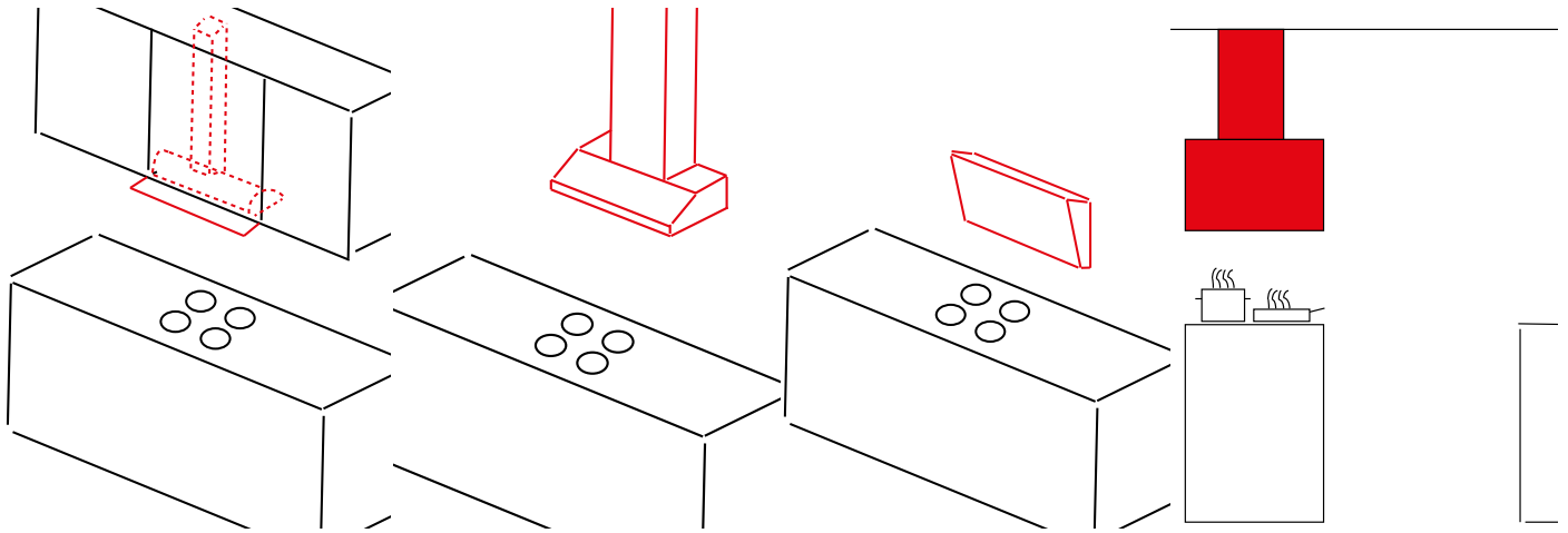
”Perinteinen” yläkaappiin asennettu liesituuletin
